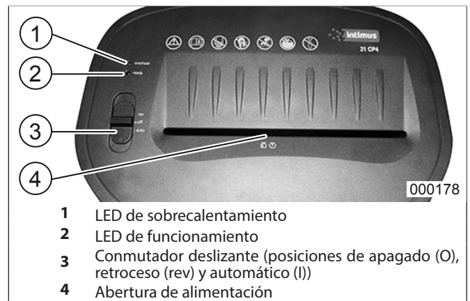
fig. 1 Elementos de mando intimus 21 CP4
