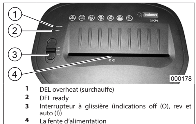
fig. 1 Elements de commande intimus 21 CP4
